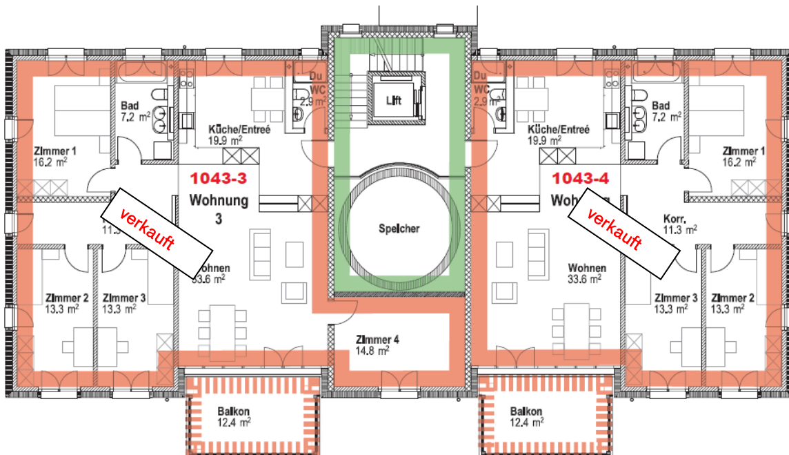
1. Obergeschoss
