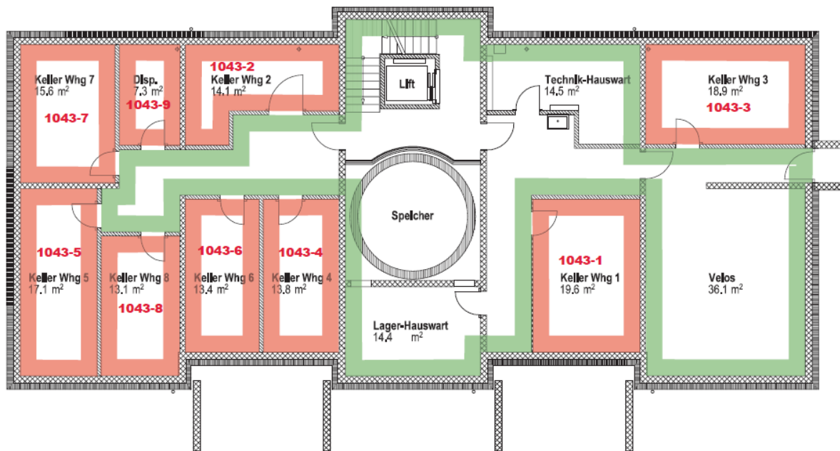
Untergeschoss
