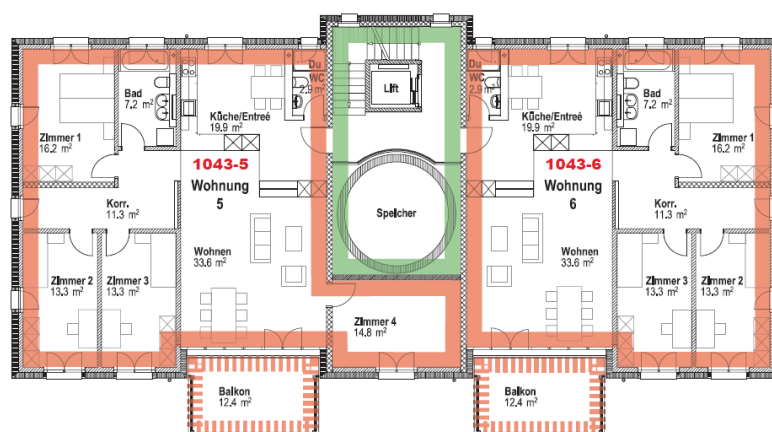
Beispiel Grundriss: 2. Obergeschoss
